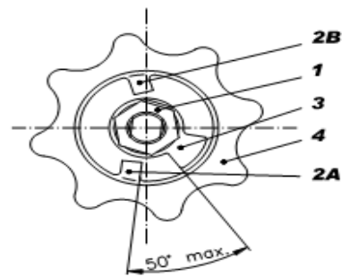
Рис. 9 Регулировка тормоза.
